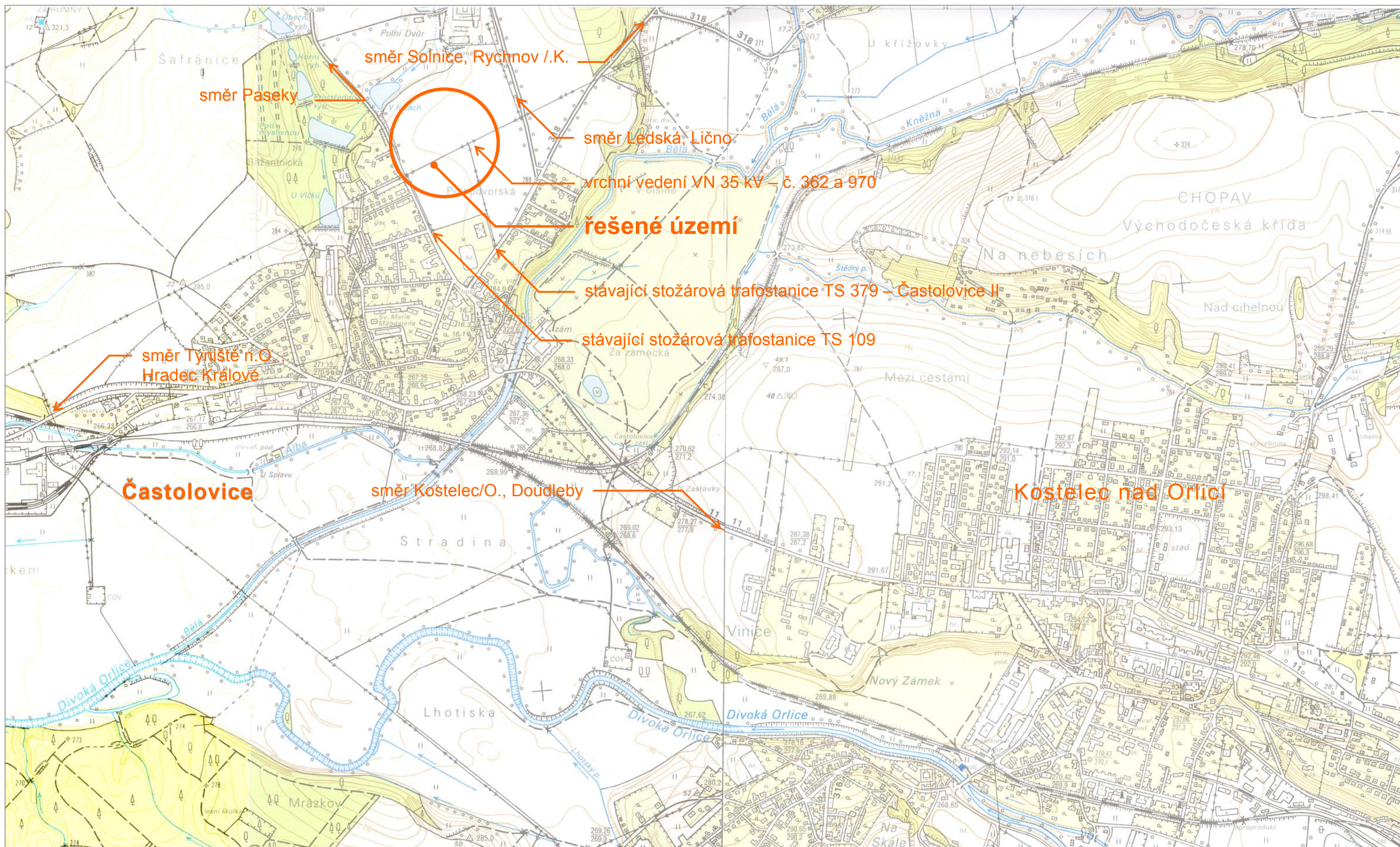
ÚZEMNÍ STUDIE • VÝSTAVBA RODINNÝCH DOMŮ ZA SOKOLOVNOU - ČASTOLOVICE • II ETAPA situace širších územních vztahů měř. 1 : 10 000 Příloha D1
