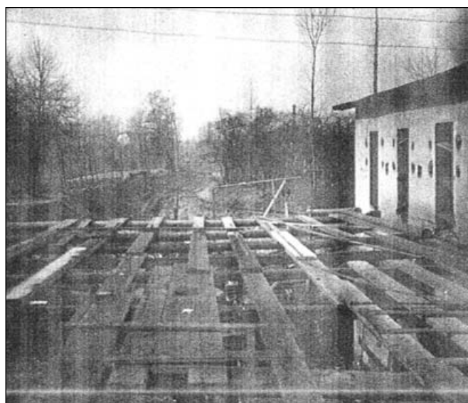
Přestavba části objektu Škopova mlýna na malou vodní elektrárnu, na podzim r. 1920.
